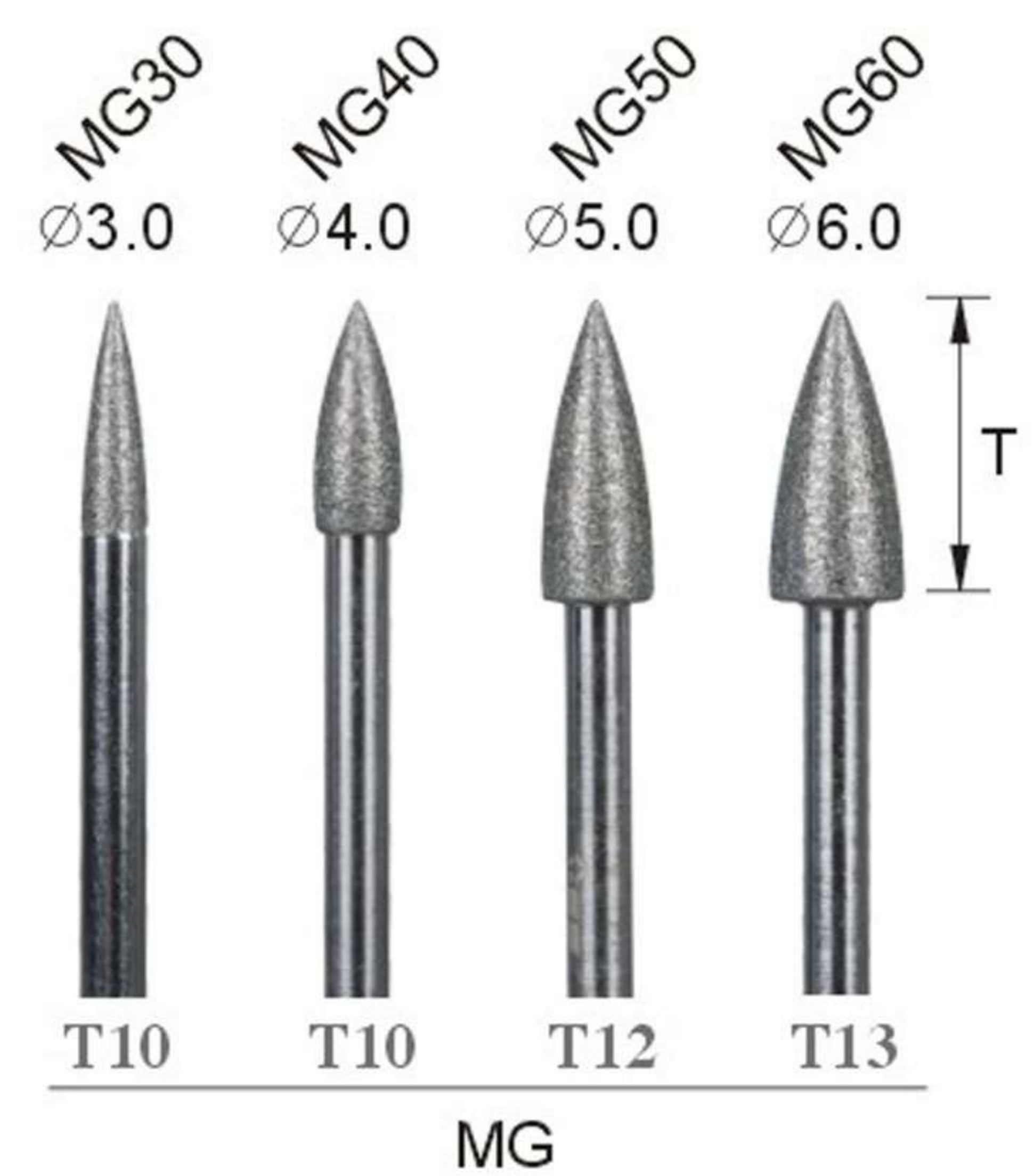
桃尖形 Needle End Taper Type
