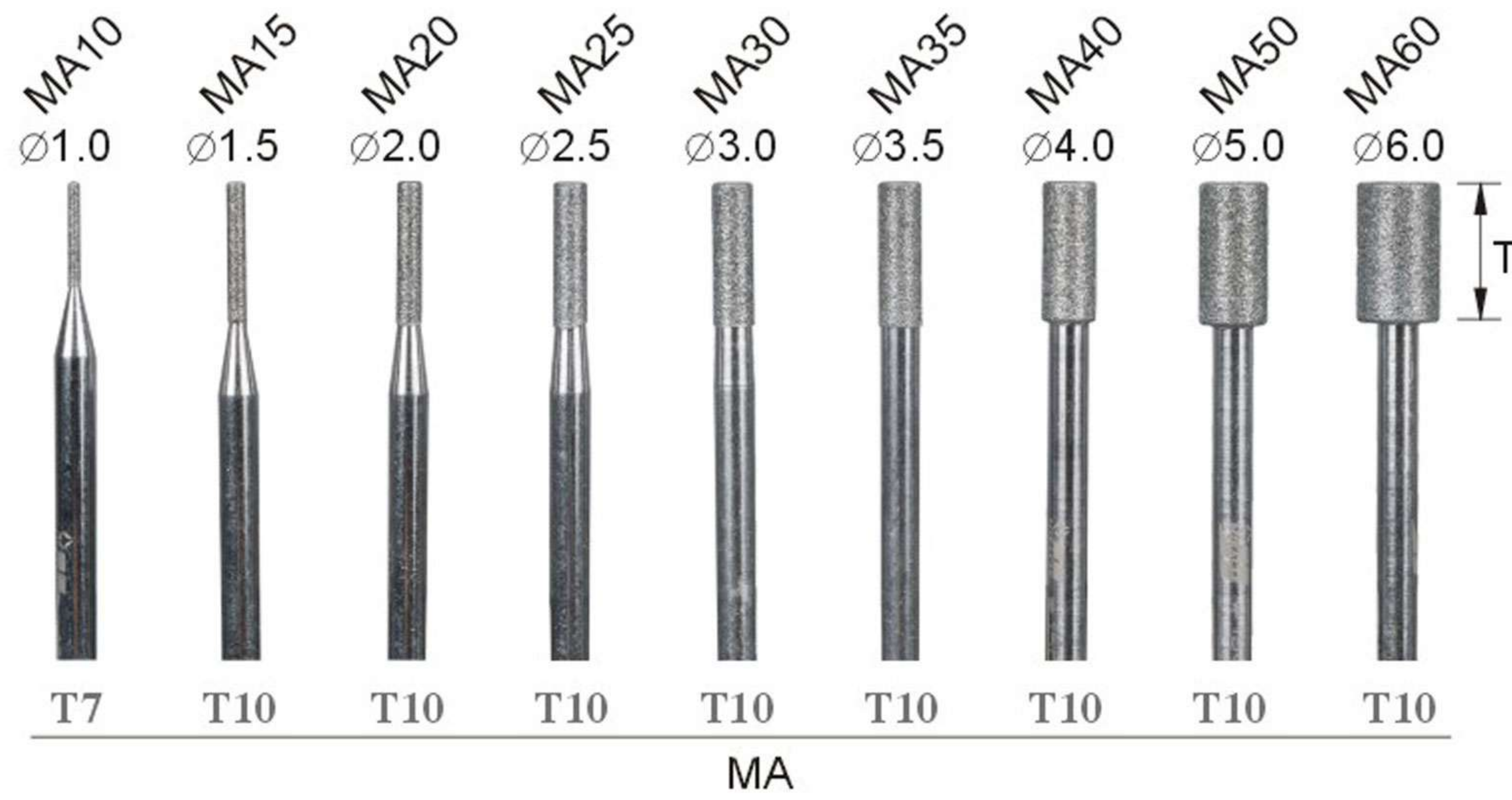
圓柱形 Cylindrical Type
