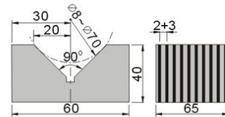
54020-04 HTV-60
