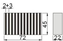
54020-03 HT-75
