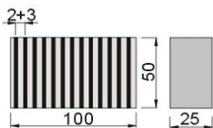
54020-05 HT-100
