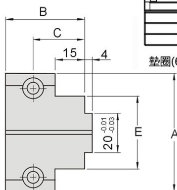
墊板、墊圈使用於 MKS-A 墊圈(64140-A)
