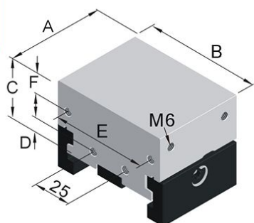
CZ固定鉗口組 CZ Fixed block
