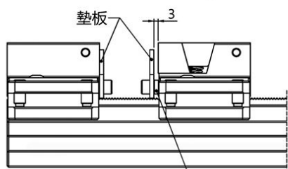
墊板、墊圈使用於 MKS-A 墊圈(64140-A)
