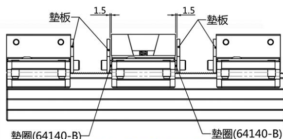
墊圈(64140-B) 墊板、墊圈使用於 MKS-B
