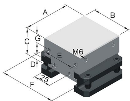
BZ固定鉗口組 BZ Fixed block
