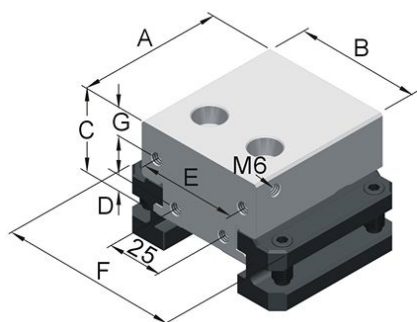
AZ固定鉗口組 AZ Fixed block
