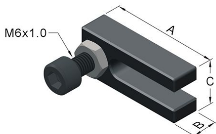
基準靠板 (M6牙) Datum Plate (M6 thread)
