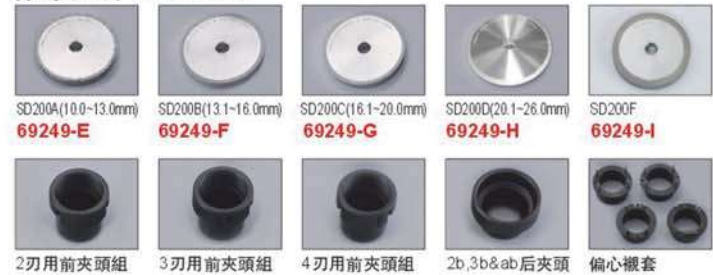
2刃用前夾頭組 3刃用前夾頭組 4刃用前夾頭組 2b,3b&ab后夾頭 偏心襯套
